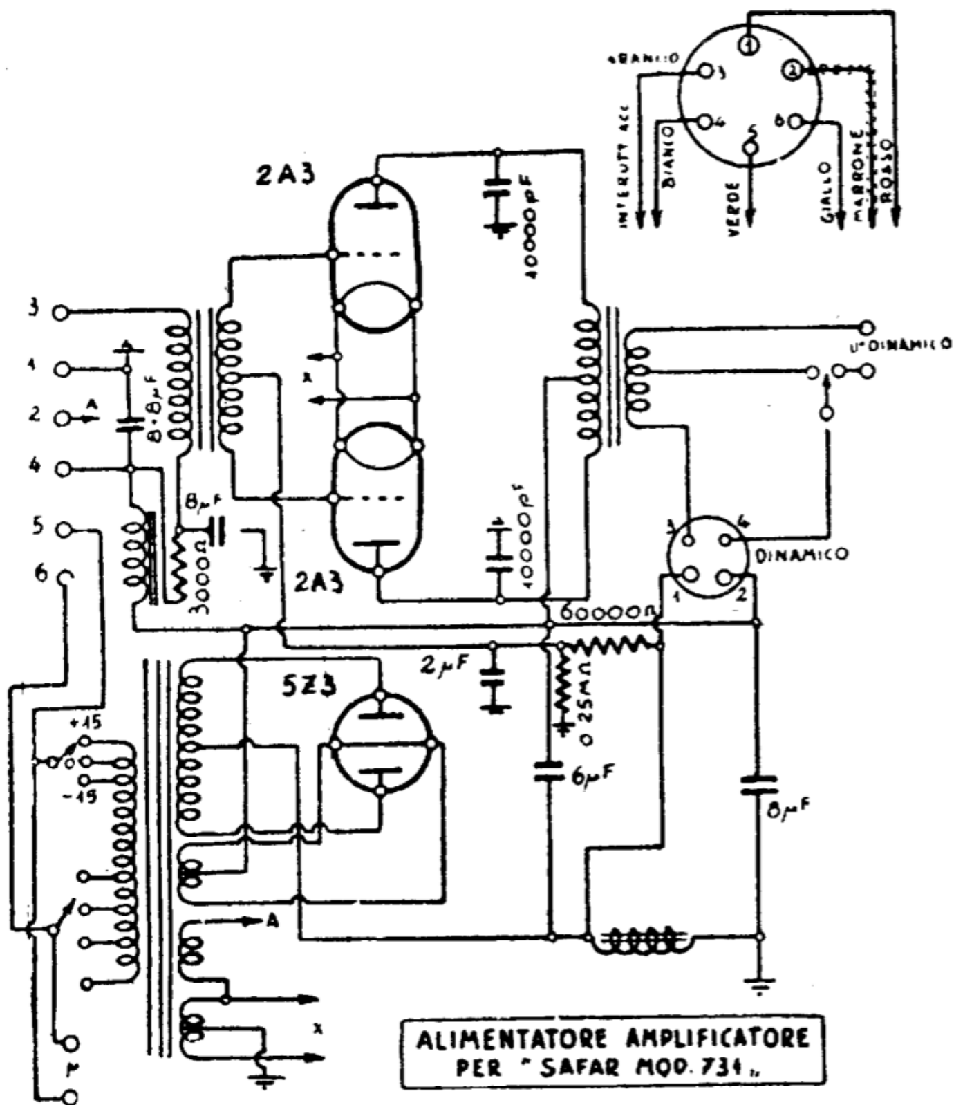
— Parte amplificatrice b. f. e parte alimentatrice del mod. « 731 » Safar.
